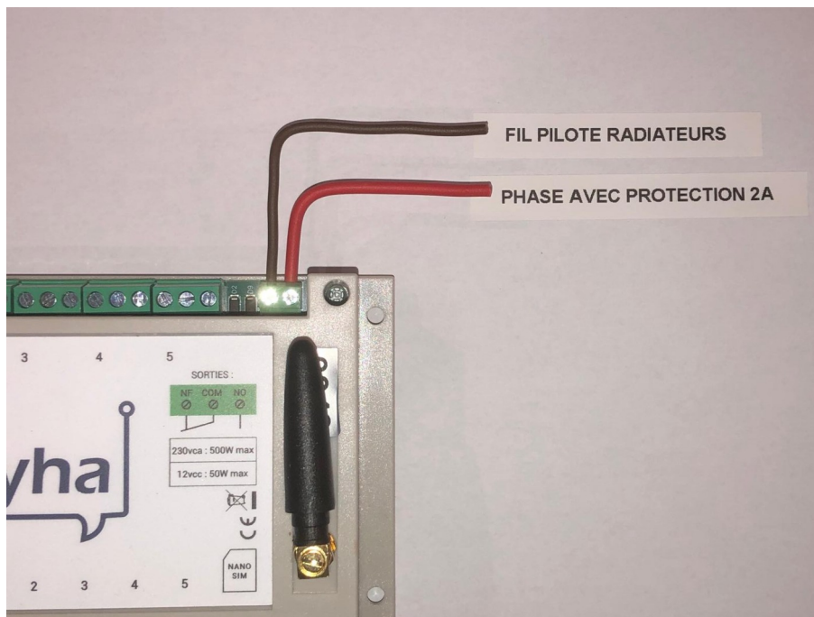
Figure 1 : Schéma de raccordement pour le fil pilote
